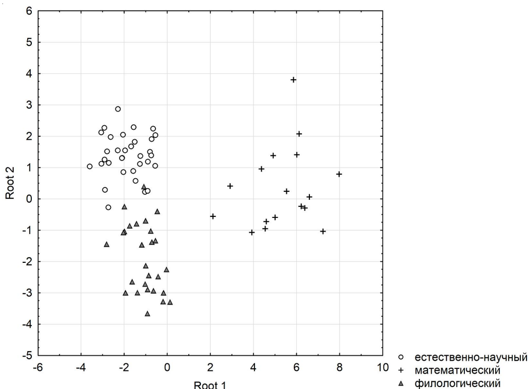
Диаграмма рассеяния канонических значений для канонических корней
